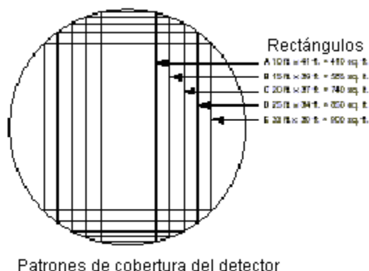
Patrones de cobertura del detector
